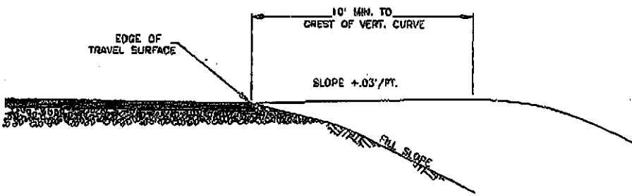
- FILL SECTION -
